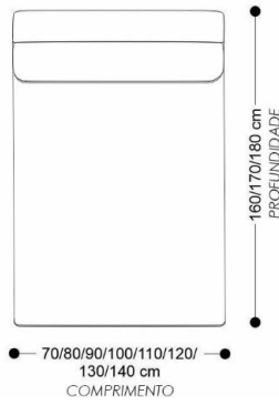
MÓDULO PUFF
